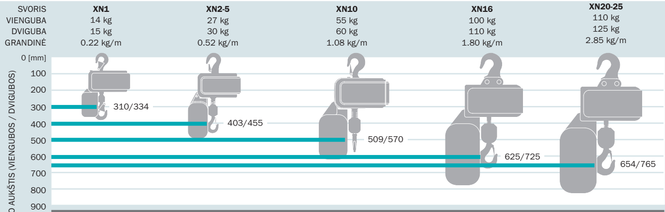
PAKĖLIMO AUKŠTIS SU SKIRTINGAIS VEŽIMĖLIŲ DERINIAIS (MM)
